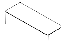
Tavolo da Pranzo 280 x 100 Dining Table 280 x 100 ABL7304 L 280cm D 100cm H 73cm L 110¼" D 39¼" H 28¾"
