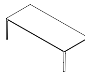
Tavolo da Pranzo 240 x 100 Dining Table 240 x 100 ABL7303 L 240cm D 100cm H 73cm L 94½" D 39¼" H 28¾"
